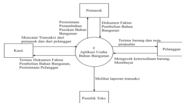
Gambar 1. Diagram Konteks
